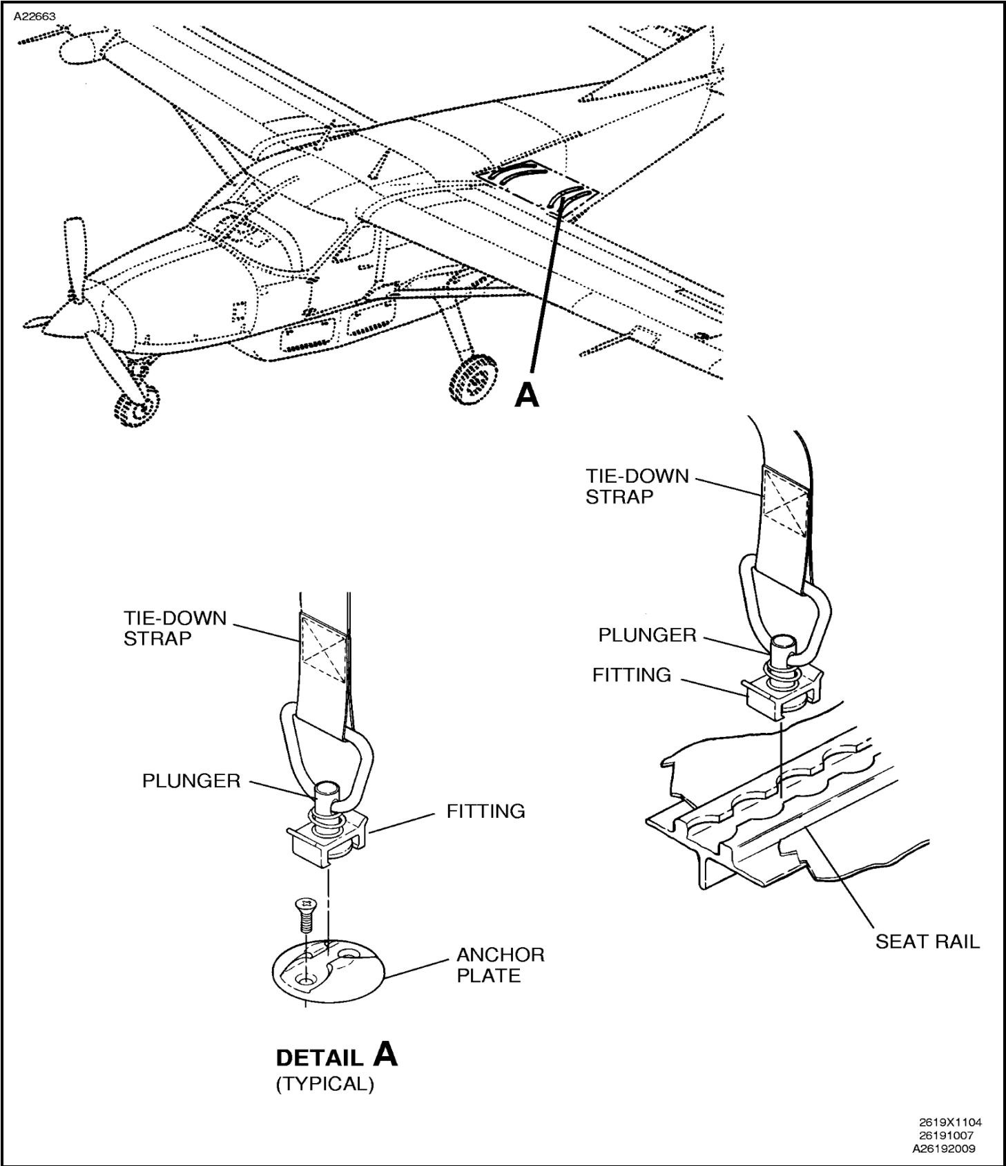
Figure 201 : Sheet 1 : Cargo Tie-Downs
